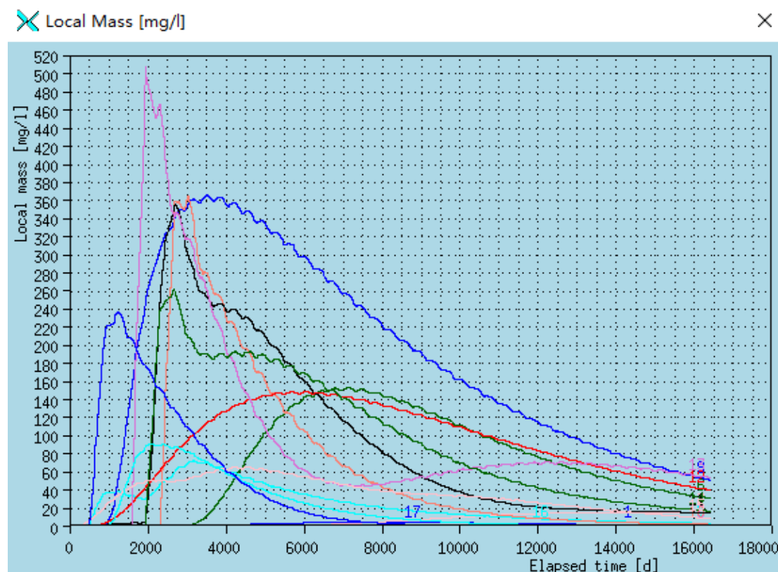
图 5.3.4-2 虎山、烂泥坑稀土矿区矿块开采镁离子浓度随时间变化曲线图
