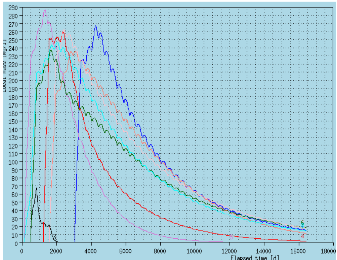
图 5.4.4-2 赤岗、窑下稀土矿区矿块开采镁离子浓度随时间变化曲线图
