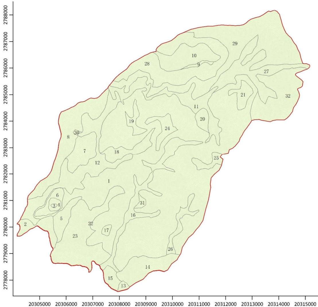
图 5.3.2-4 虎山、烂泥坑模拟区含水层渗透系数分区
