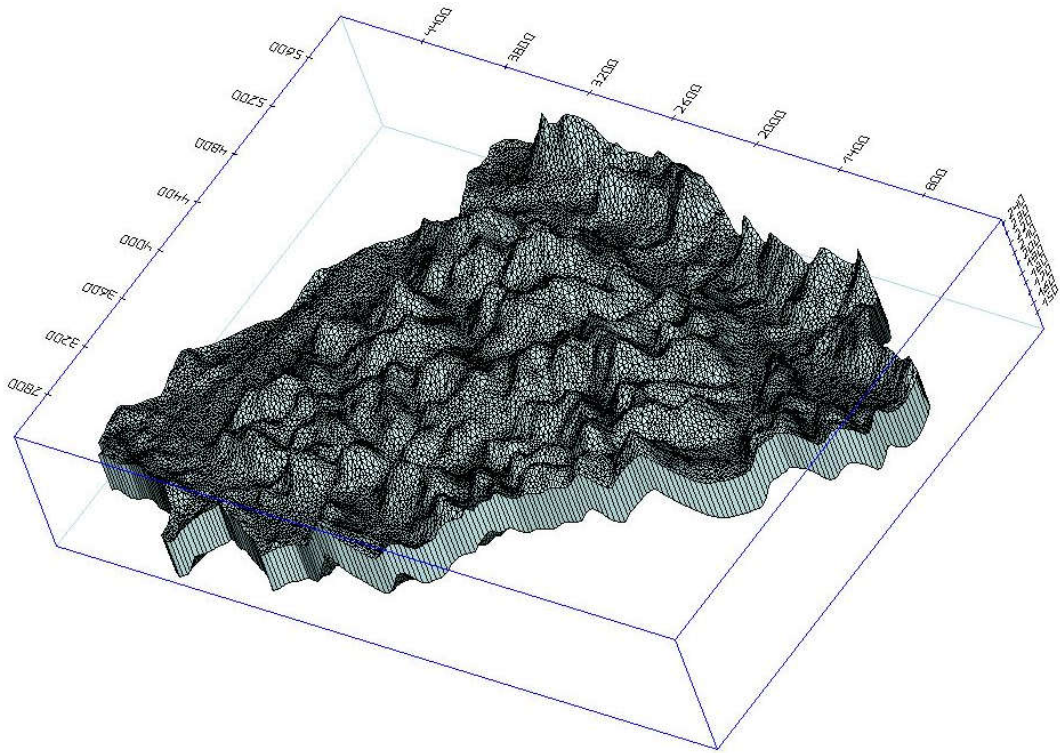
图 5.2.2-2 地下水渗流模型的网格剖分立体图
