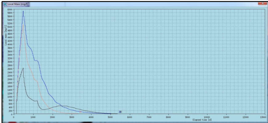
图 5.2.4-4 安西矿区矿块开采硫酸根离子浓度随时间变化曲线
