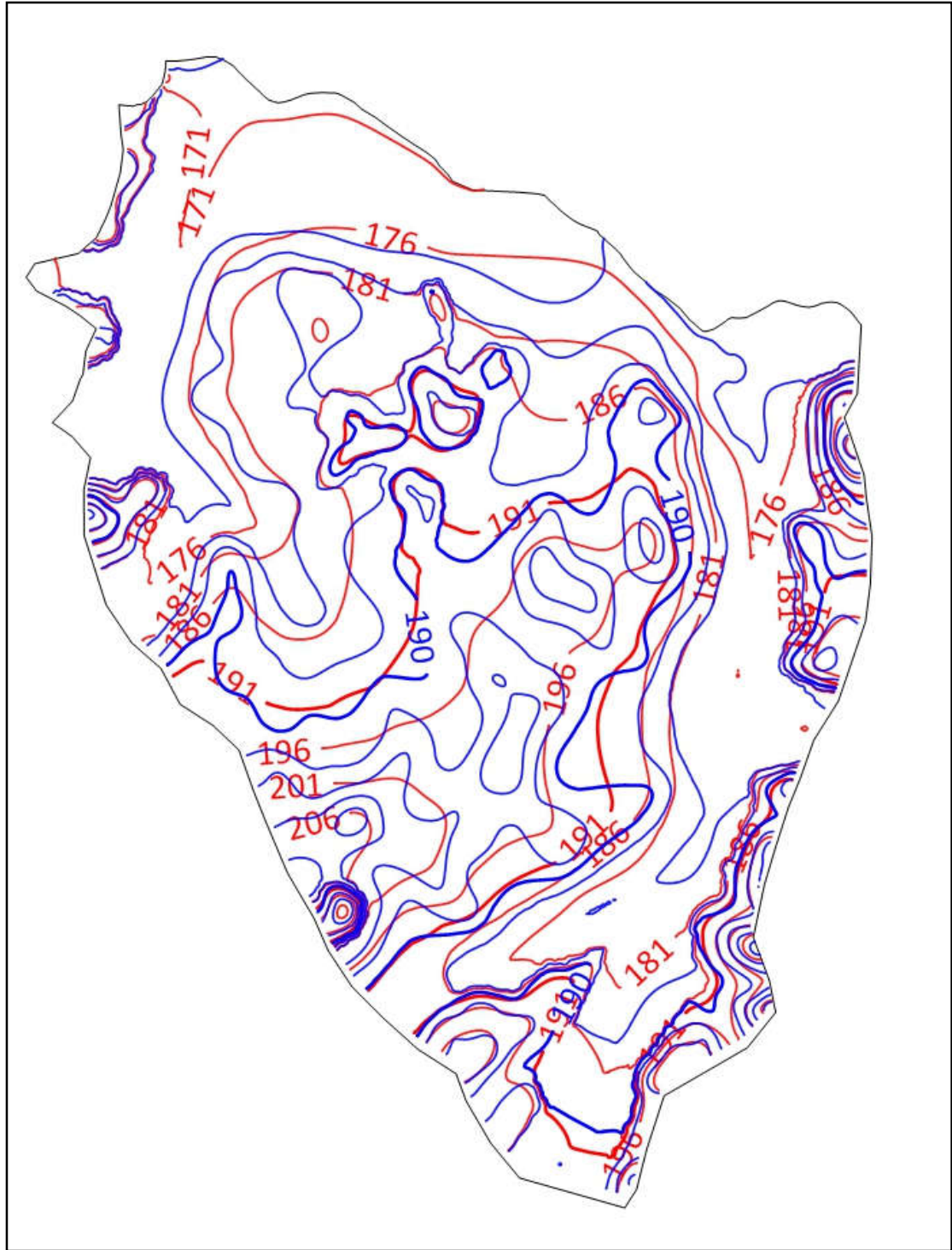
图 5.2.2-6 模拟区枯水期实测等水位线与计算等水位线对比图 (2021.11)
