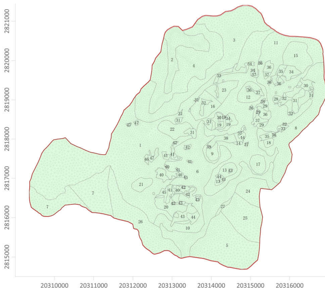
图 5.4.2-3 赤岗、窑下模拟区降雨入渗系数分区
