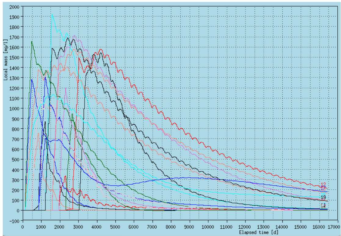
图 5.4.4-4 赤岗、窑下稀土矿区矿块开采硫酸根离子浓度随时间变化曲线
