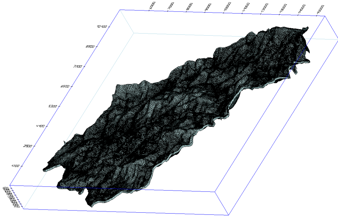
图 5.3.2-2 地下水渗流模型的网格剖分立体图
