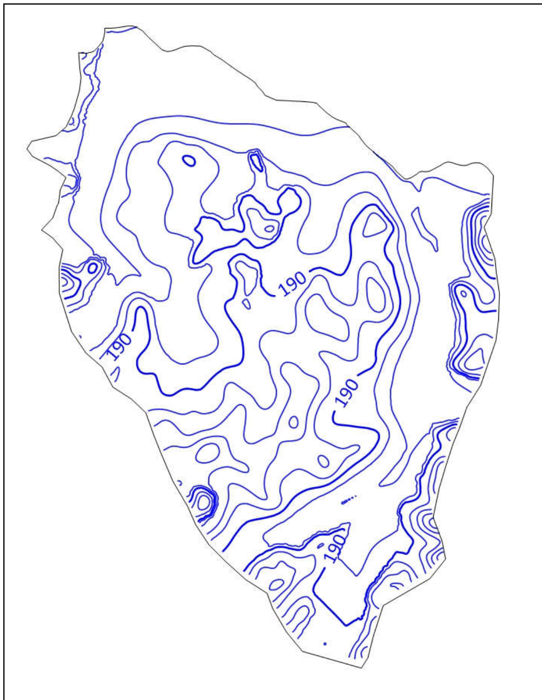
图 5.2.2-5 初始水位等值线图（2021.8）
