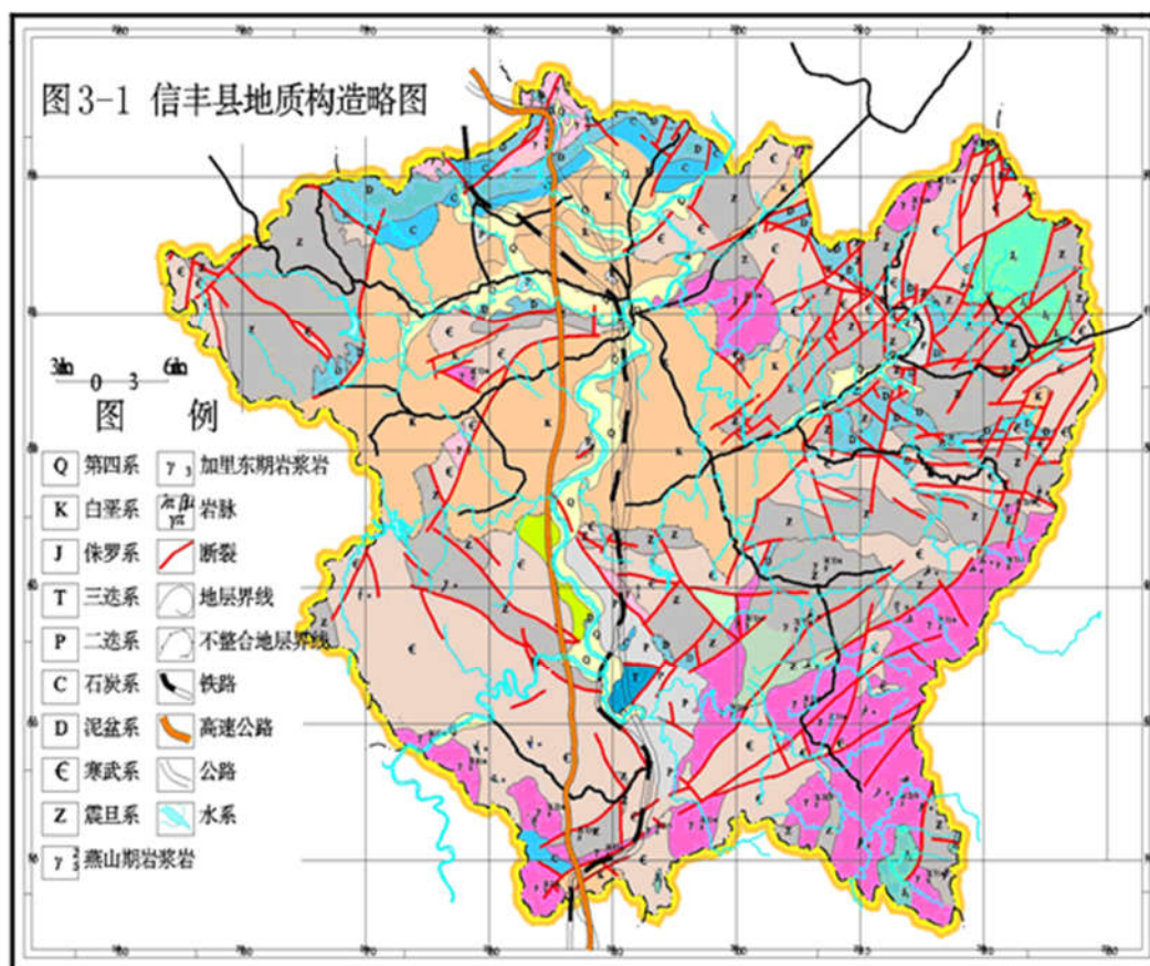
图 2.4.1-1 地质构造
