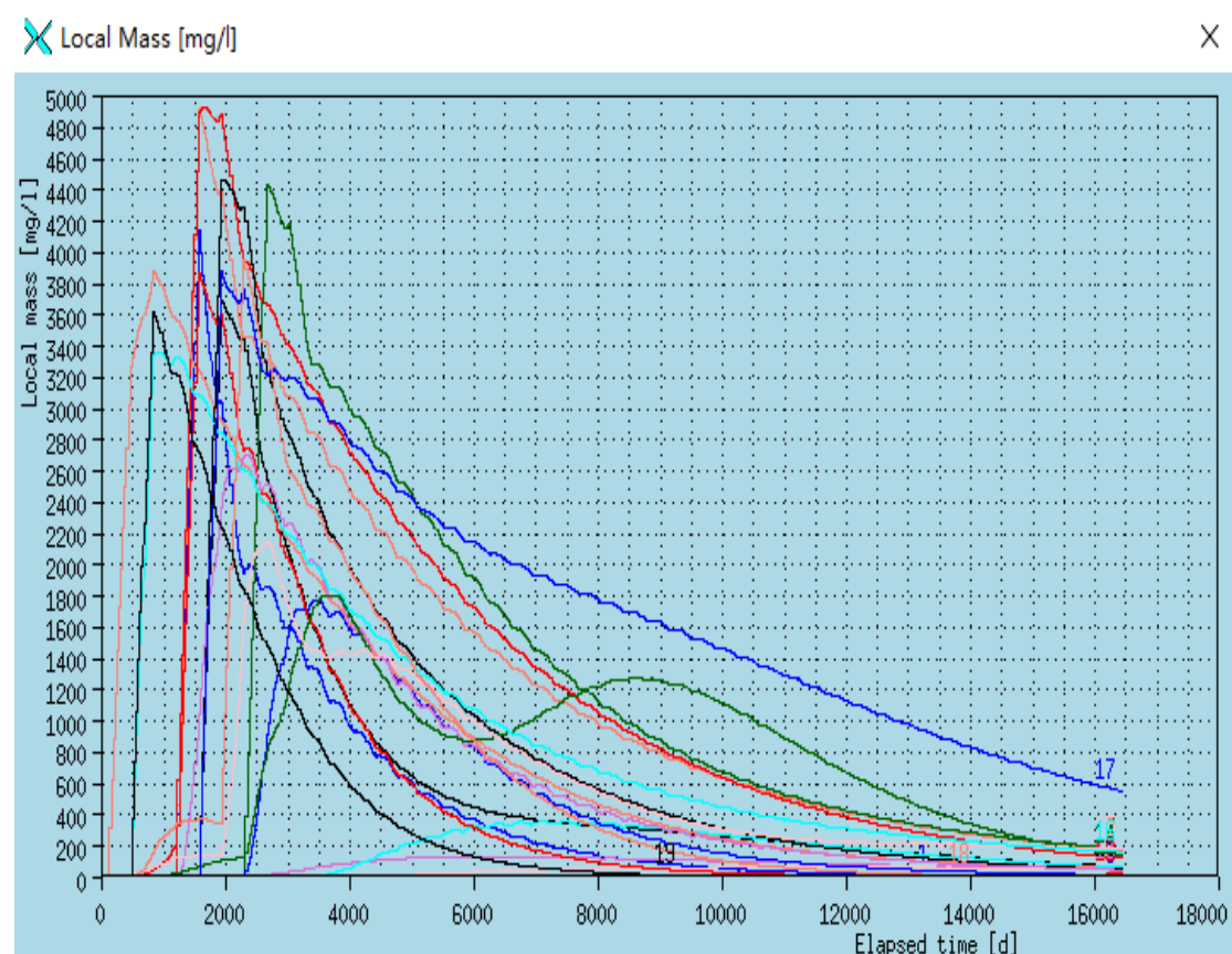
图 5.3.4-4 虎山、烂泥坑稀土矿区矿块开采硫酸根离子浓度随时间变化曲线
