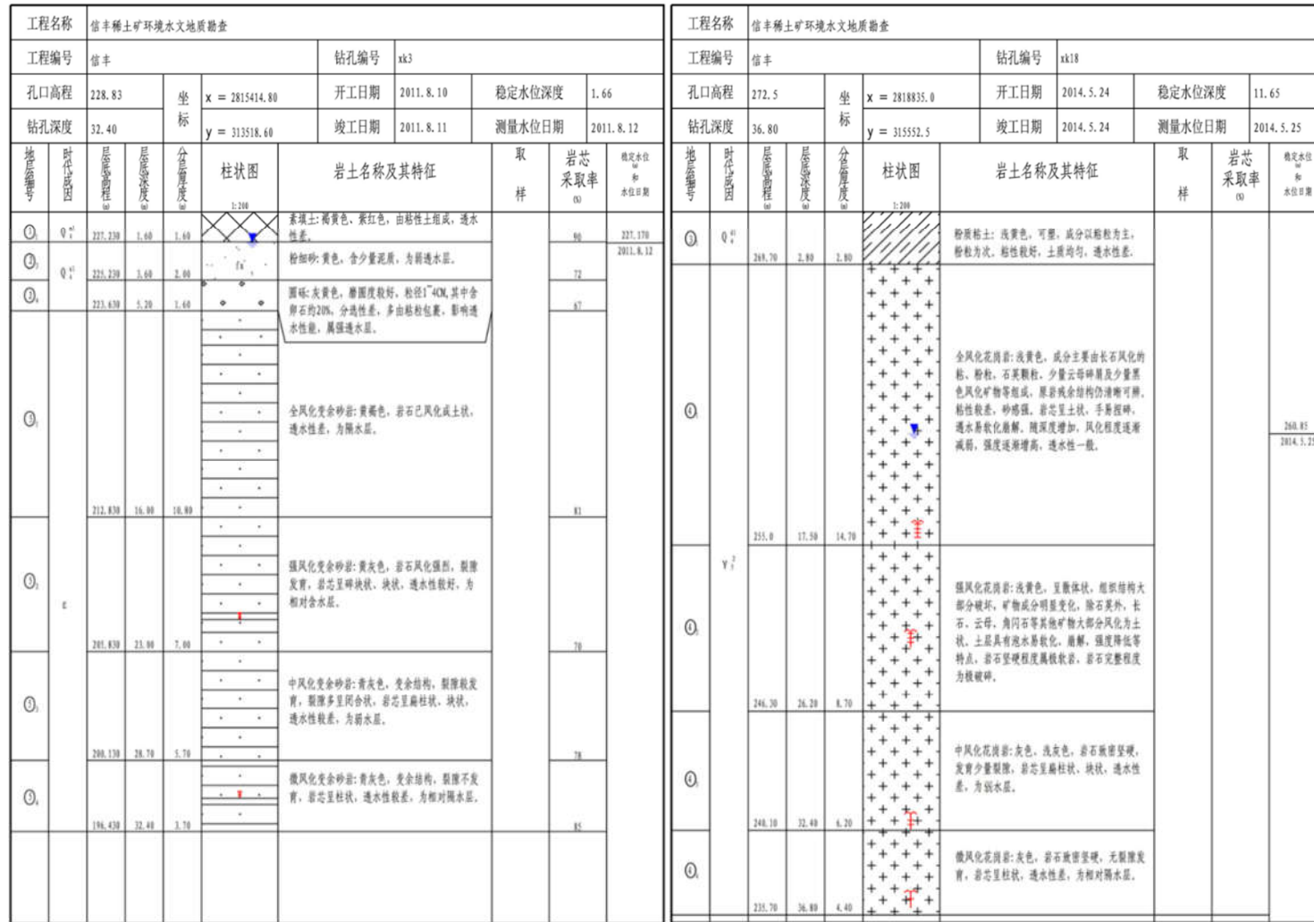
图 3.3.2-1 信丰赤岗、窑下、赣县韩坊稀土矿环境水文地质勘查钻孔柱状图
