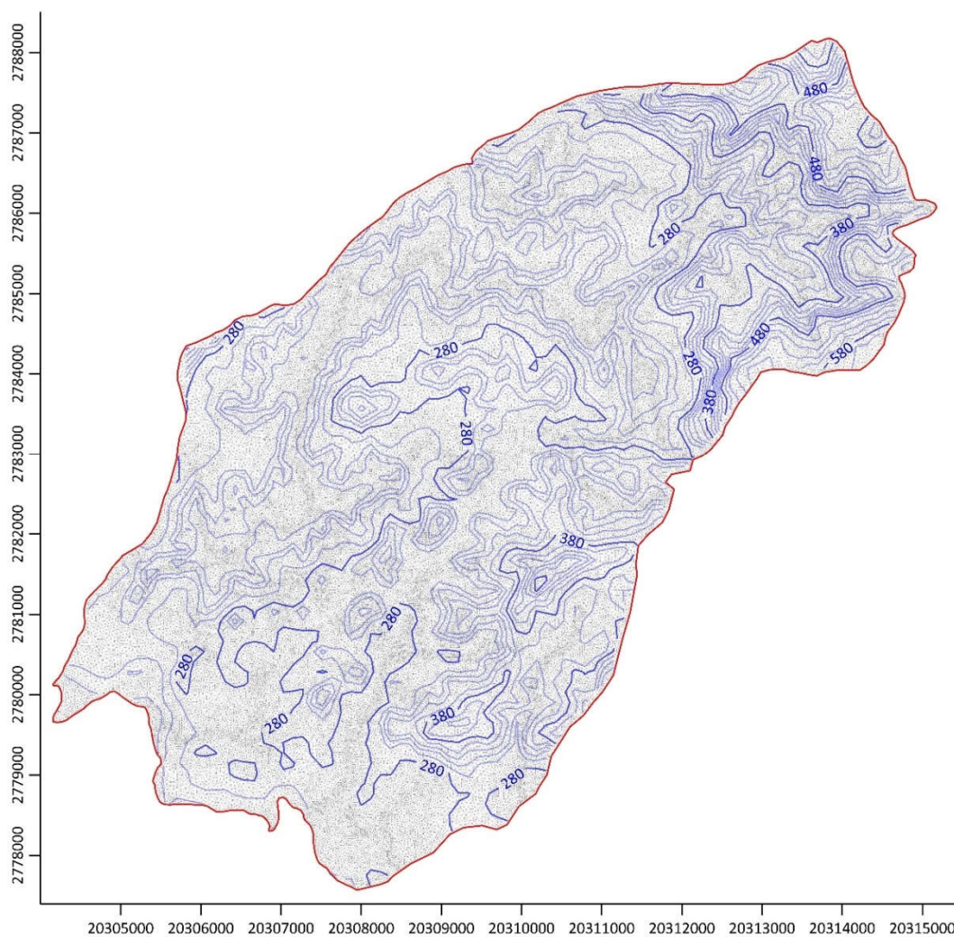
图 5.3.2-5 初始水位等值线图 (2021.8)
