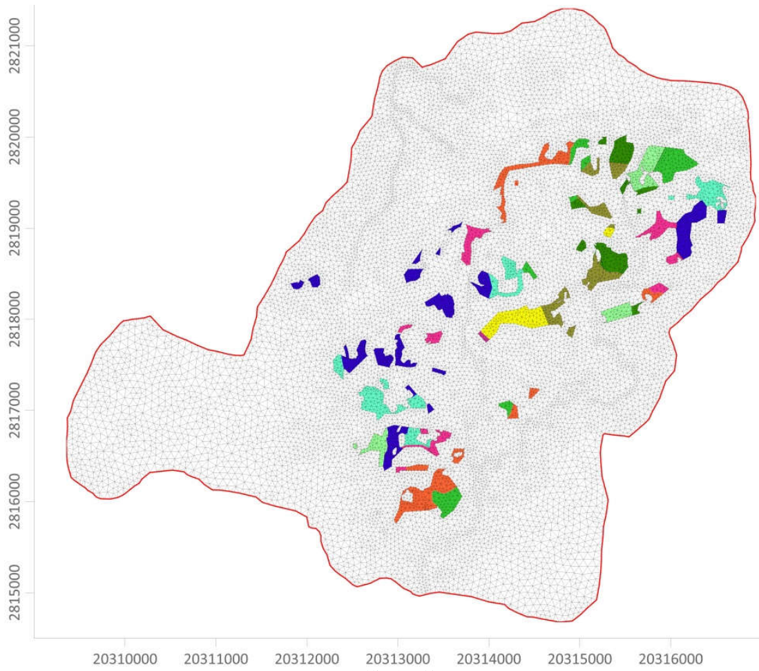
图 5.4.2-1 模型网格剖分图
