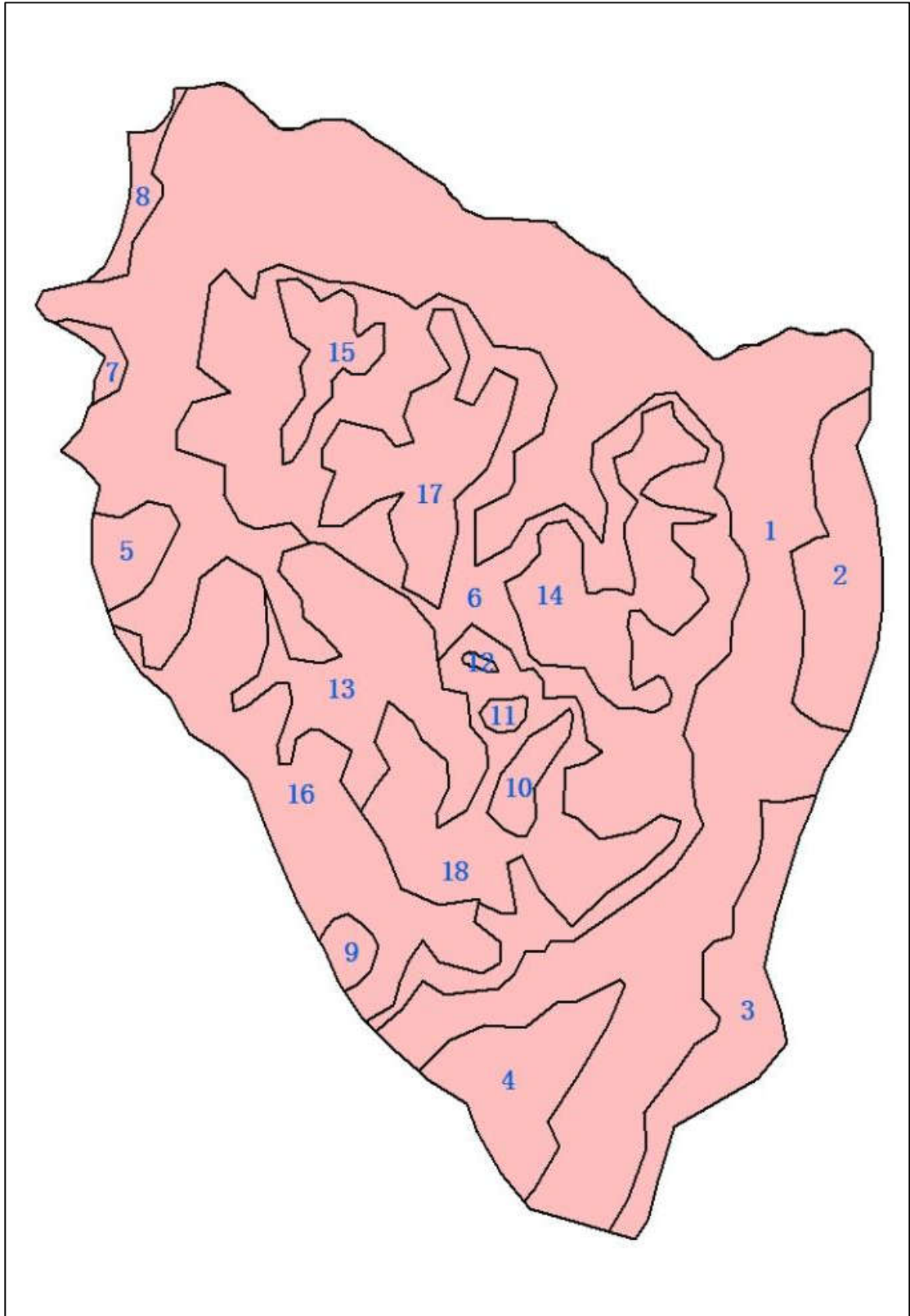
图 5.2.2-4 安西模拟区含水层渗透系数分区
