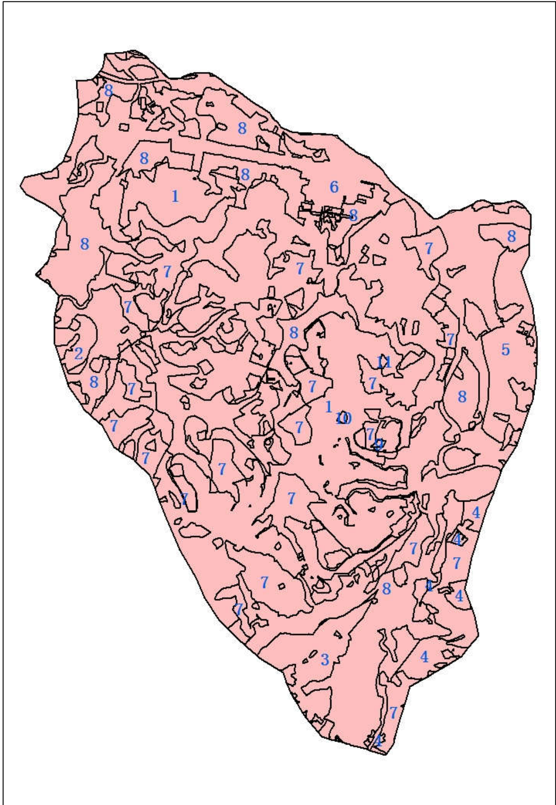
图 5.2.2-3 安西模拟区降雨入渗系数分区
